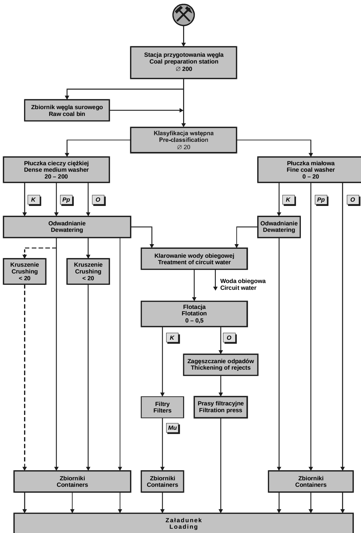
Rys. 3 Schemat blokowy zakładu przeróbczego KWK Marcel
