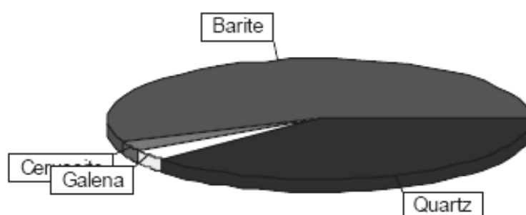
Rys. 6 Skład mineralogiczny próbki z okolic Kraslic
